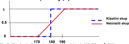
Slika. Grafički prikaz klasičnog i neizrazitog skupa za varijablu: visoki ljudi (Izvor: Čerić, Varga, 2004, str. 177)
